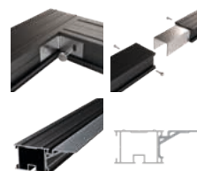
Profiel P418
