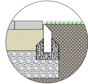
Plaatsingsmodel
